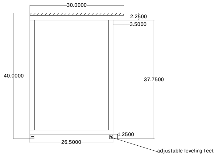
End Elevation
